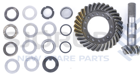
Carraro Kron spidshjuls sæt CNH, Komatsu, Caterpillar
